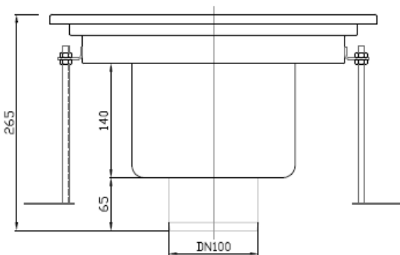
Zij aanzicht
