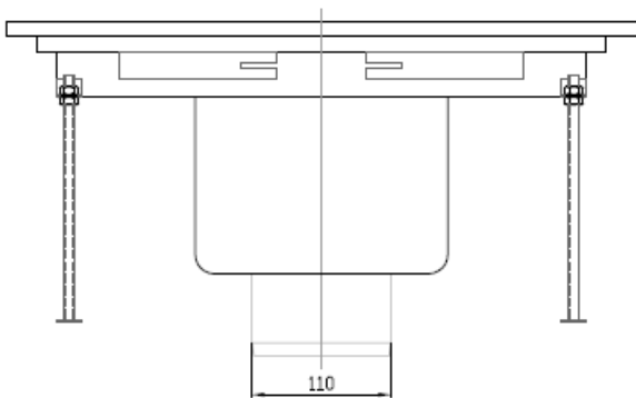
Front aanzicht
